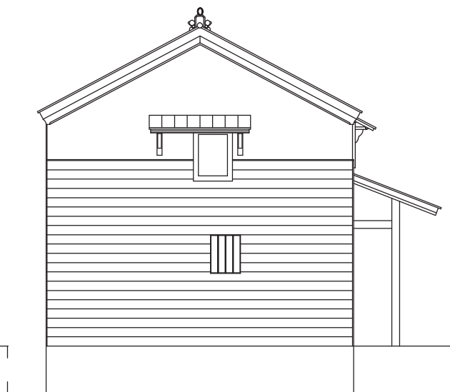
南側立面図
